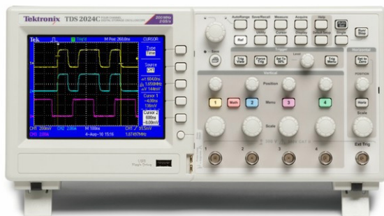
Obr. 2. Digitální osciloskop Tektronix TDS 2024C
