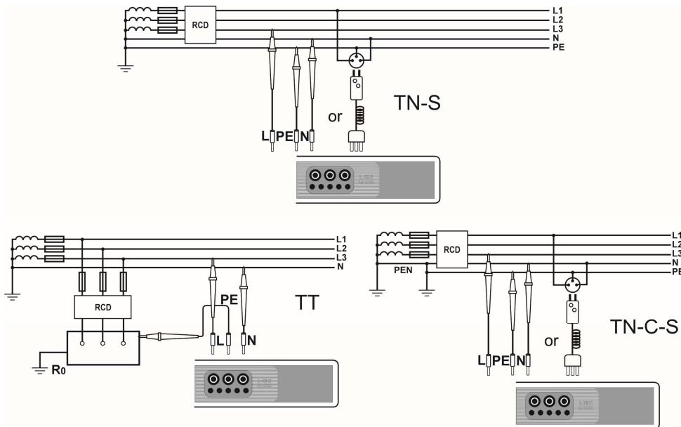
Měření v systémech TN, TT
